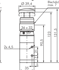
3/2-Wege Not-Aus-Taster
