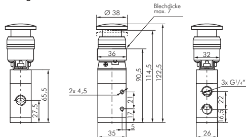
3/2-Wege Pilztaster
