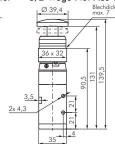
5/2-Wege Not-Aus-Taster
