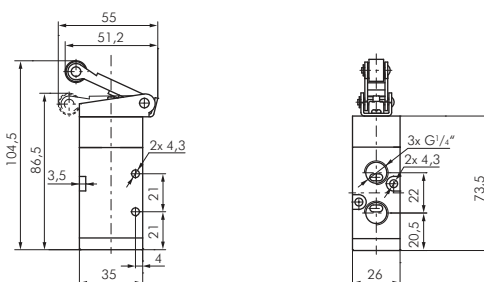
5/2-Wege Rollenhebelventil
