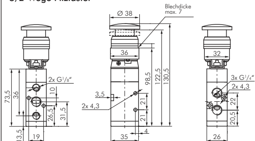
5/2-Wege Pilztaster
