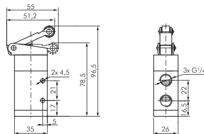
3/2-Wege Rollenhebelventil
