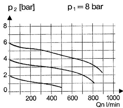
5.6. Durchflusscharakteristik
