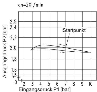
5.7. Hysterese
