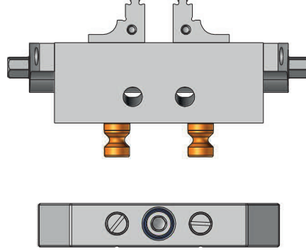
Product Nr. 2316 Pull Stud
